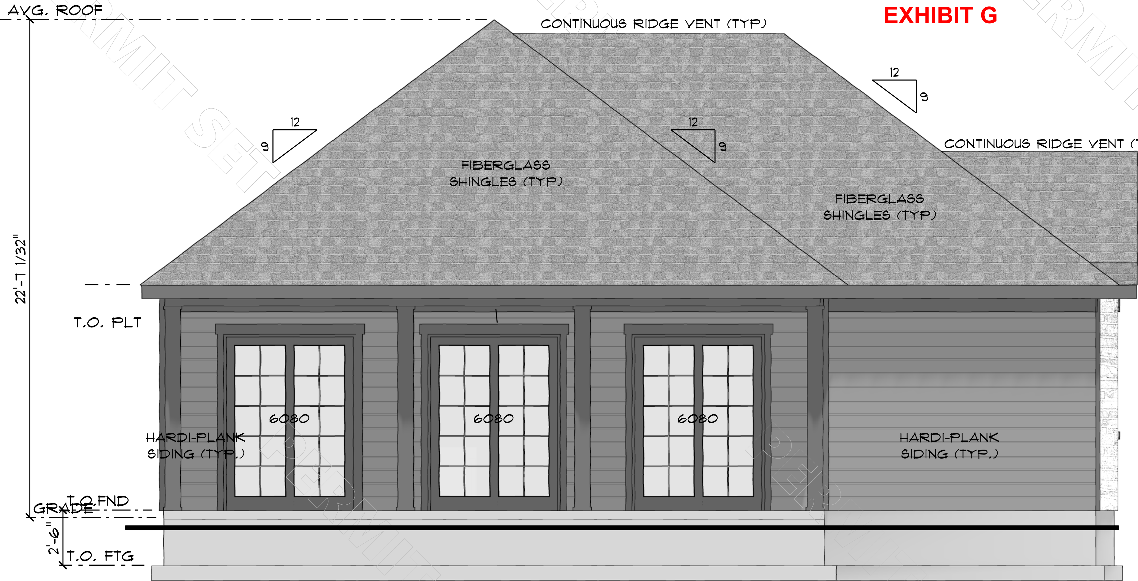
FRONT ELEVATION SCALE: 3/8" = 1'-0"
