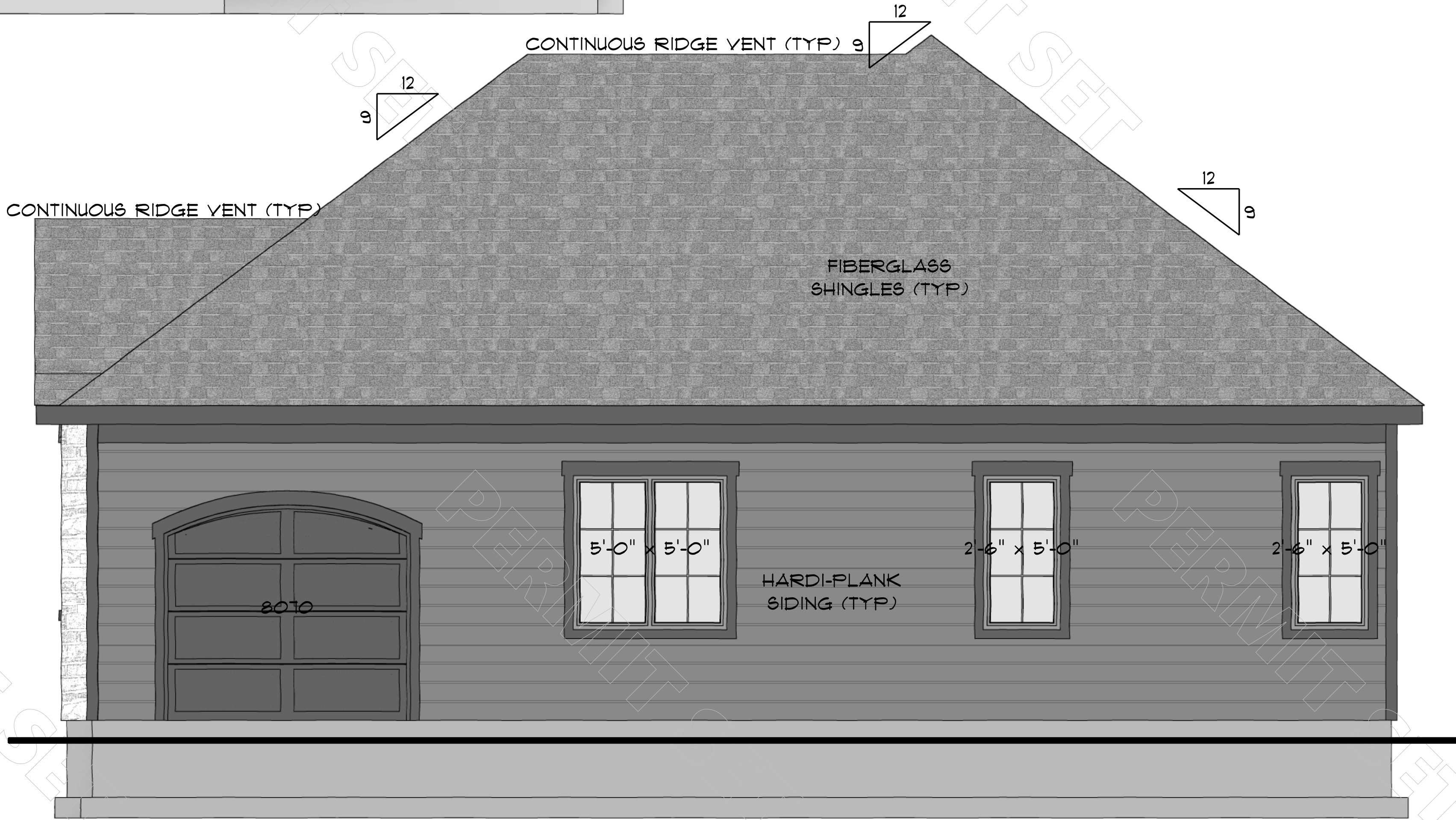
REAR ELEVATION SCALE: 3/8" = 1'-0"
