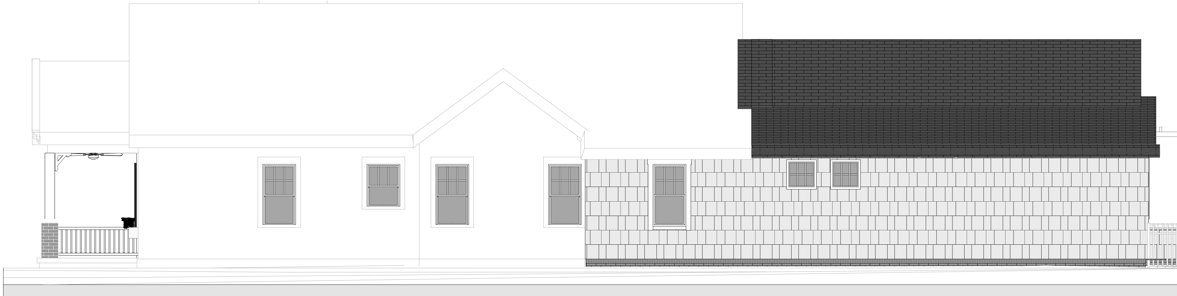
1 A5 Front or WEST ELEVATION SCALE: 1/4" = 1'-0"
