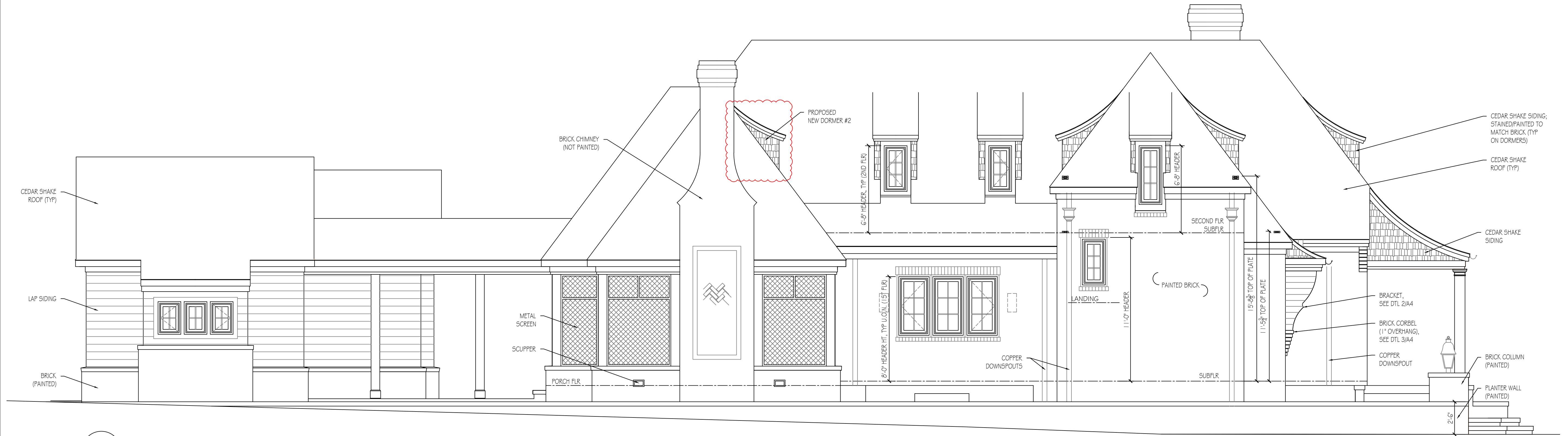
1 EAST ELEVATION A11 SCALE: 1/4" = 1'-0"
