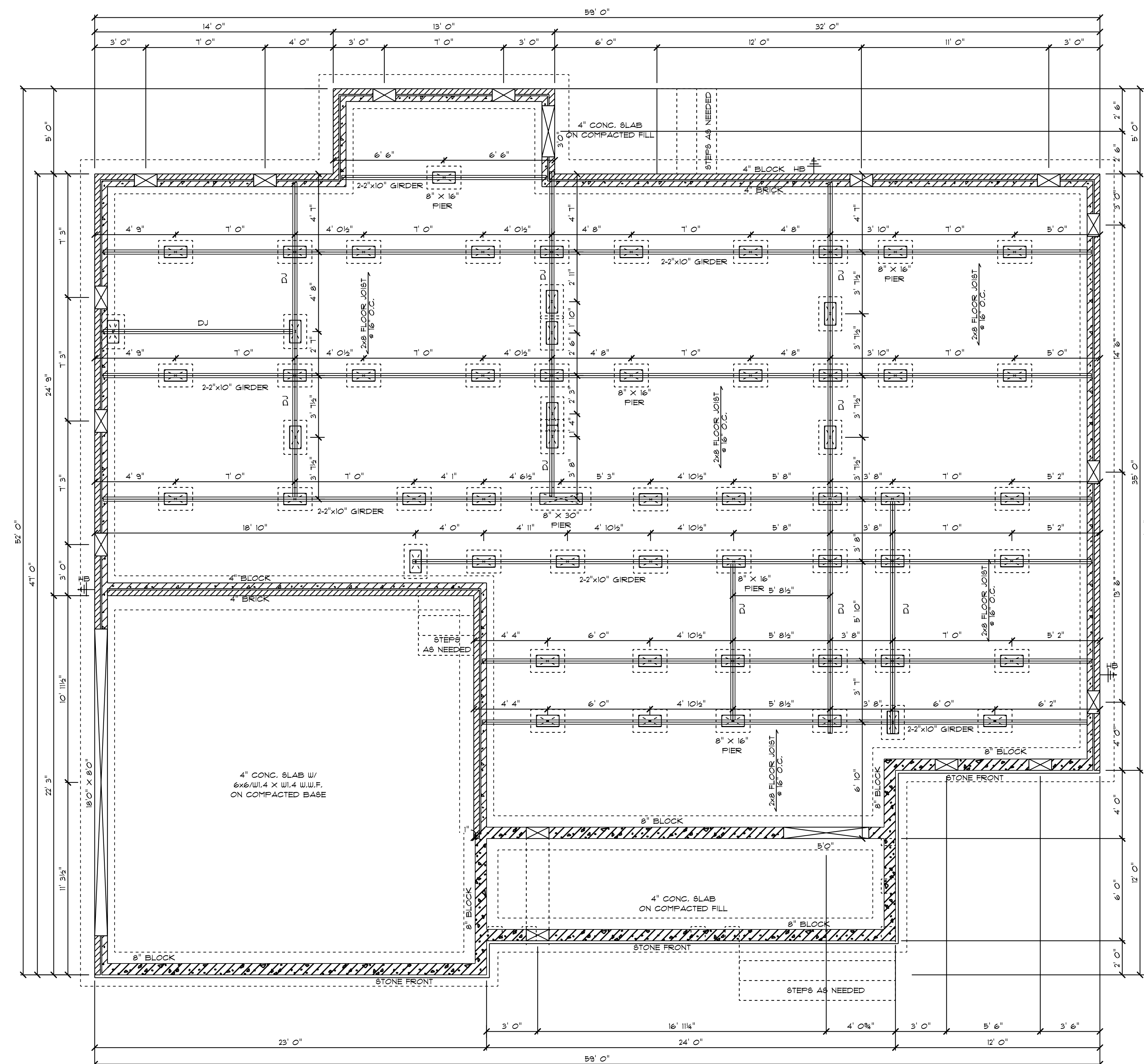
CRAWLSPACE FOUNDATION SCALE: 1/4" = 1'0"
