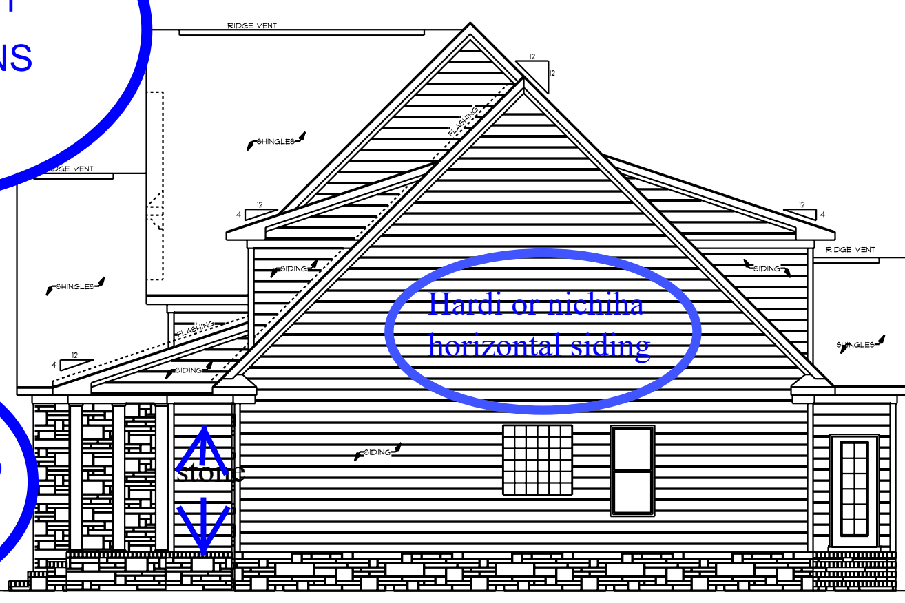
RIGHT ELEVATION SCALE: 1/8" = 1'
