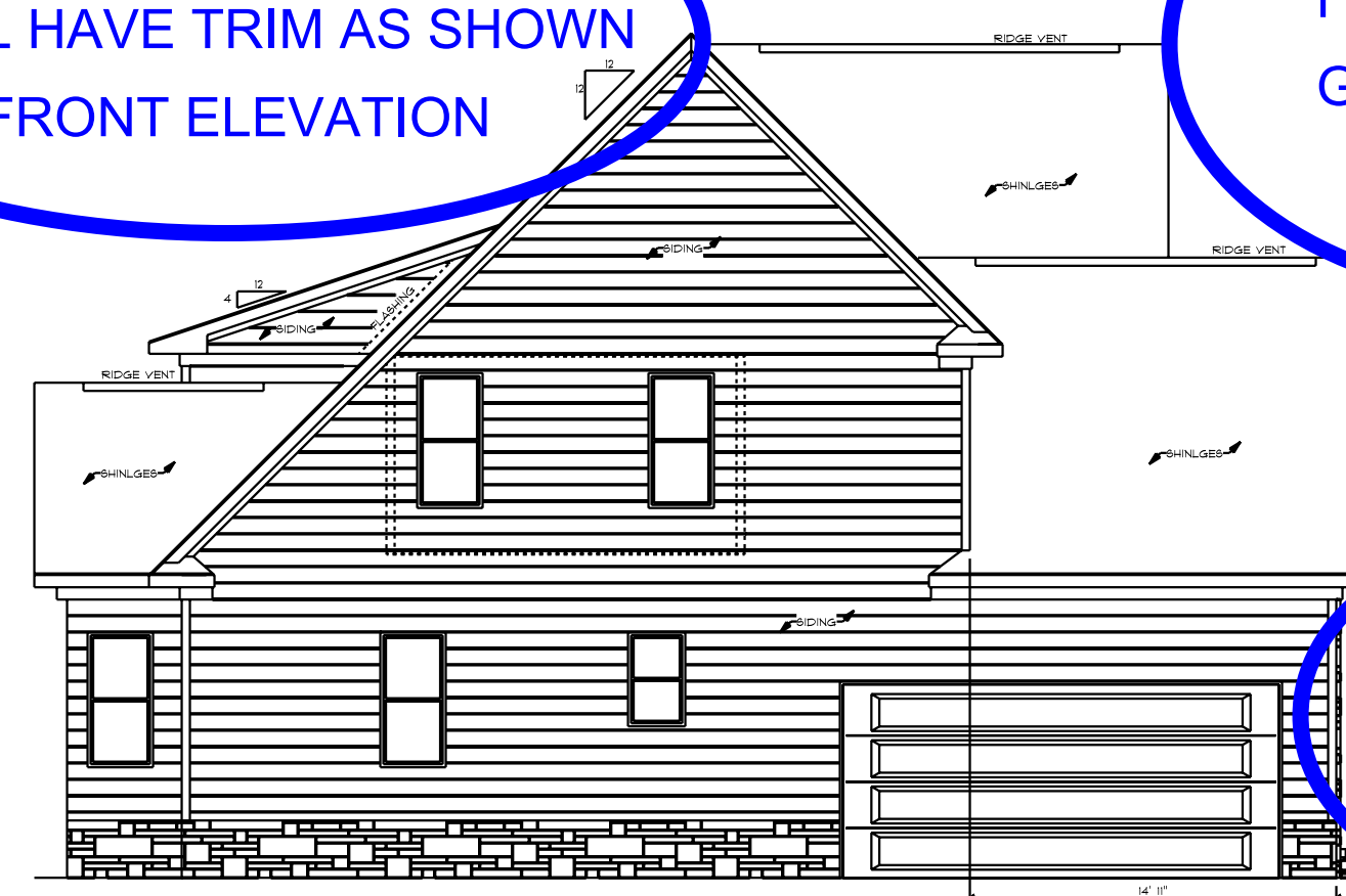
LEFT ELEVATION SCALE: 1/8" = 1'
