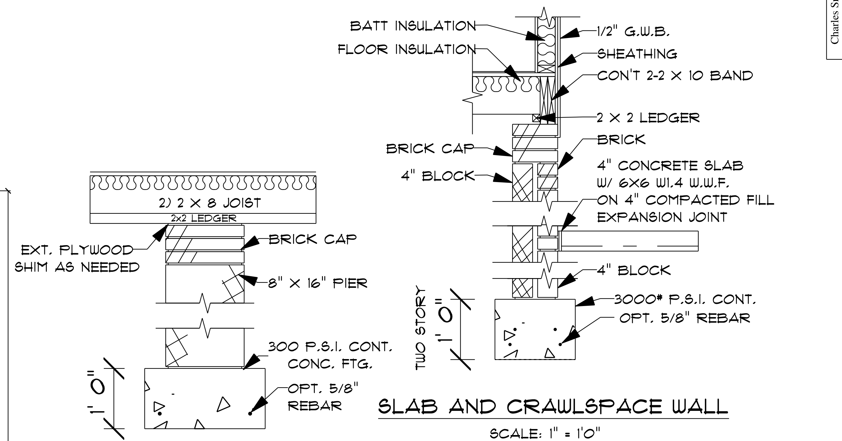
DOUBLE JOIST PIER SCALE: 1" = 1'0"
